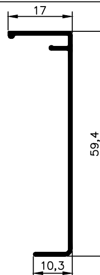
NX 5809 0,245 Kg/m
