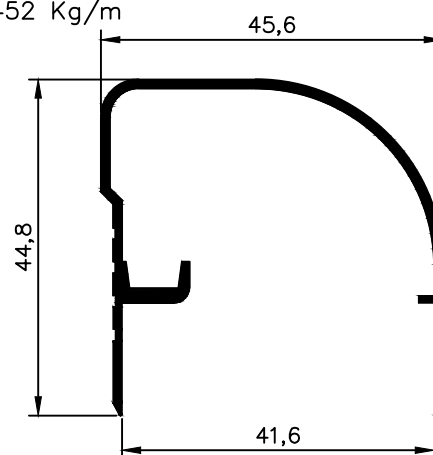
NX 6464 0,452 Kg/m
