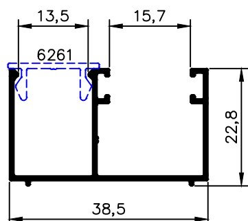
NX 6262 0,288 Kg/m
