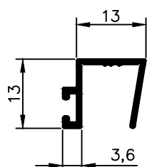
NX 6044 0,125 Kg/m
