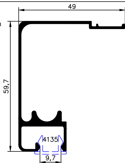
NX 5908 0,606 Kg/m
