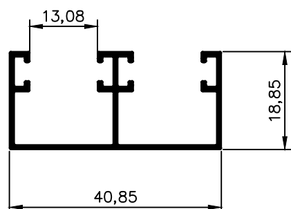
NX 5998 0,320 kg/m
