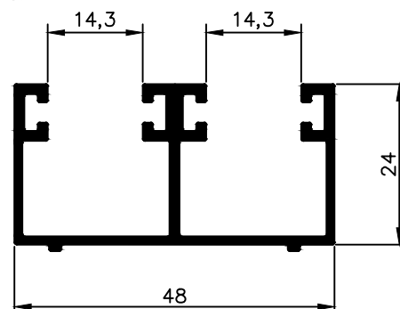
NX 4125 0,598 Kg/m
