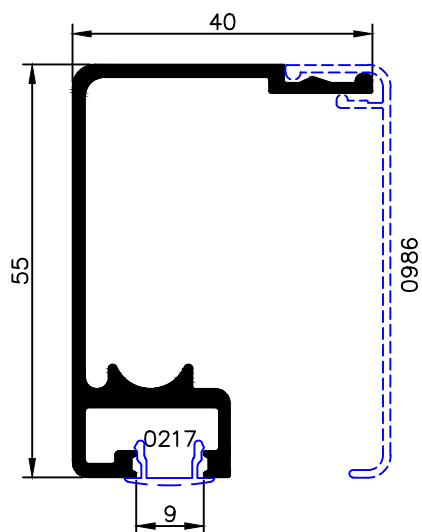
NX 0984 0,701 Kg/m
