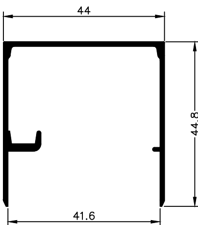
NX 0628 0,505 Kg/m
