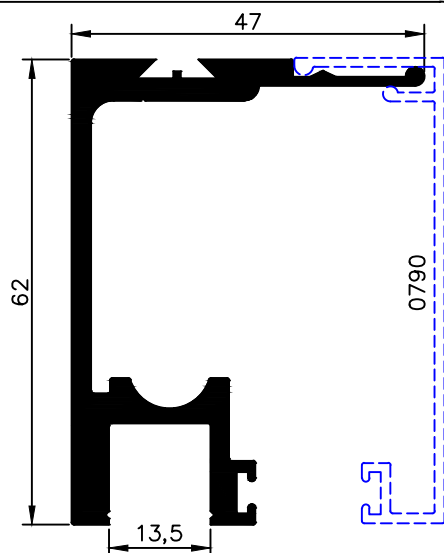
NX 0789 1,272 Kg/m
