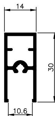
NX 0779 0,316 Kg/m
