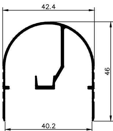
NX 1557 0,504 Kg/m
