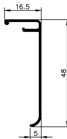
NX 0214 0,208 Kg/m
