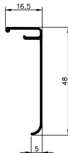
NX 0214 0,208 Kg/m
