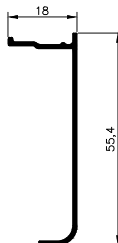
NX 5978 0,244 Kg/m
