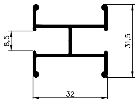
NX 3792 0,433 Kg/m
