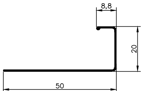
NX 4467 0,209 Kg/m
