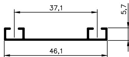
NX 4630 0,150 Kg/m
