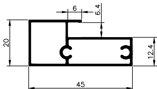
NX 4518 0,421 Kg/m
