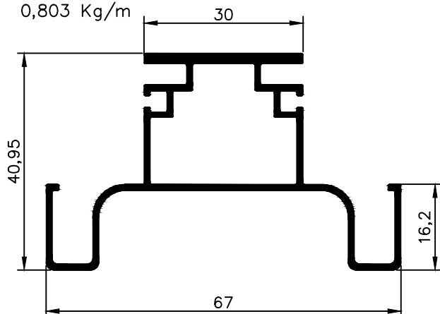
NX 3864 0,803 Kg/m
