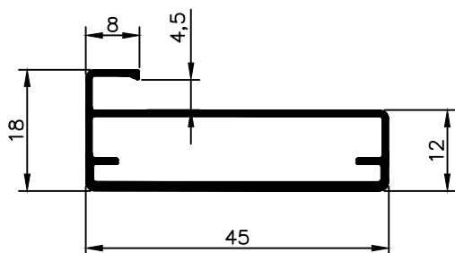
NX 2835 0,401 Kg/m
