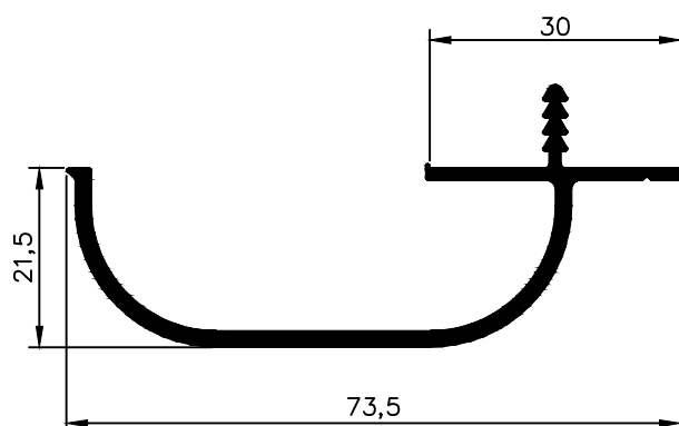
NX 2562 0,635 Kg/m
