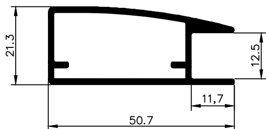
NX 0410 0,645 Kg/m
