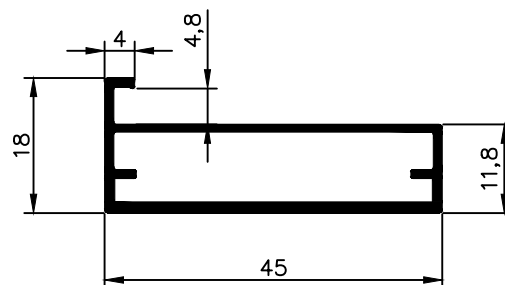
NX 4055 0,416 Kg/m
