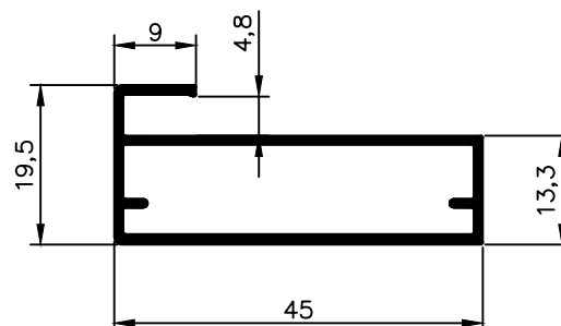
NX 4979 0,422 Kg/m
