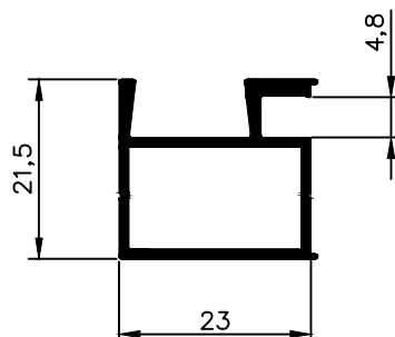
NX 2238 0,324 Kg/m
