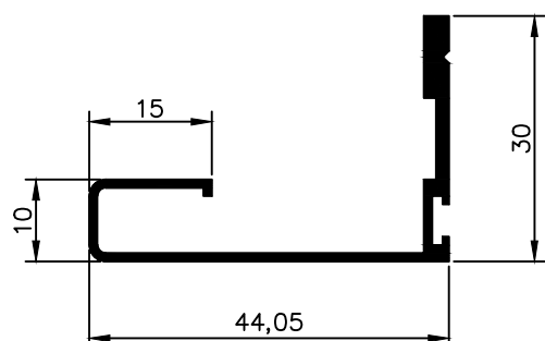
NX 1522 0,350 Kg/m
