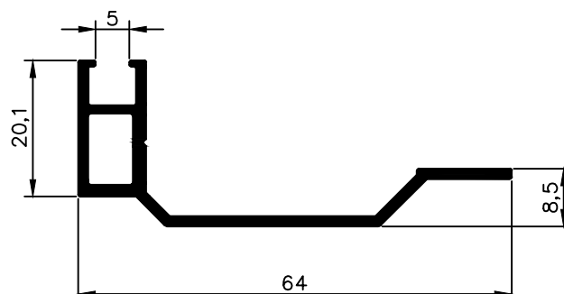
NX 3492 0,481 Kg/m
