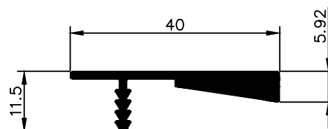
NX 4675 0,381 Kg/m
