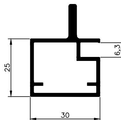
NX 4295 0,630 Kg/m
