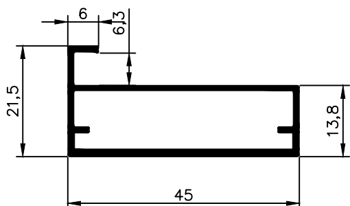
NX 2986 0,441 Kg/m
