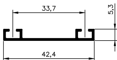
NX 2866 0,180 Kg/m
