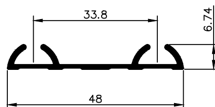
NX 4350 0,249 Kg/m
