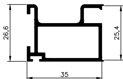
NX 2351 0,559 Kg/m
