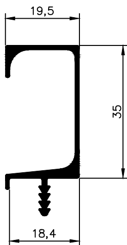
NX 4488 0,382 Kg/m
