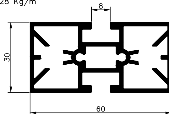
NX 1333 1,428 Kg/m
