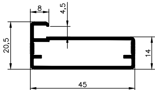
NX 3907 0,504 Kg/m
