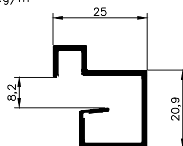
NX 2175 0,331 Kg/m
