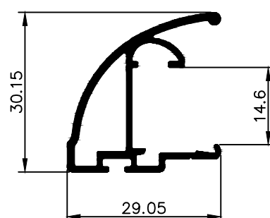
NX 4015 0,406 Kg/m
