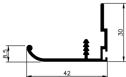
NX 2431 0,382 Kg/m
