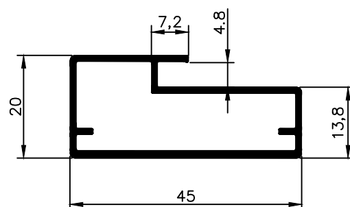
NX 2170 0,482 Kg/m
