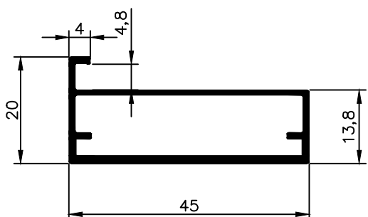
NX 2163 0,428 Kg/m
