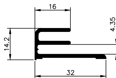
NX 0870 0,297 Kg/m
