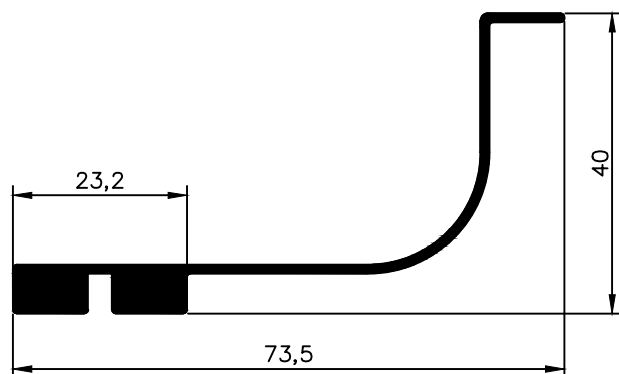
NX 1904 0,612 Kg/m
