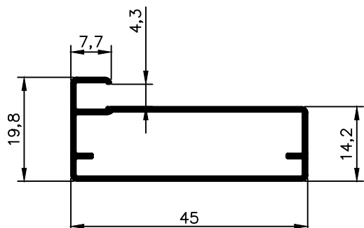
NX 6021 0,359 Kg/m
