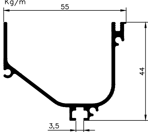
NX 3812 0,587 Kg/m
