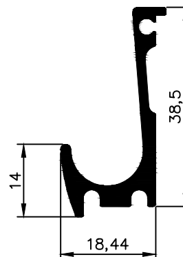
NX 2895 0,470 Kg/m
