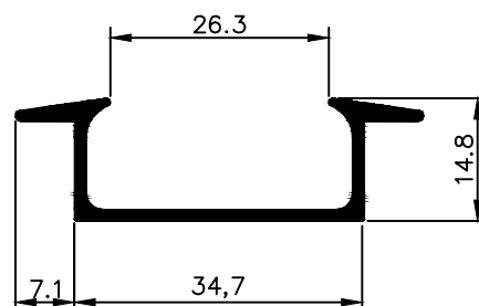
NX 2484 0,336 Kg/m
