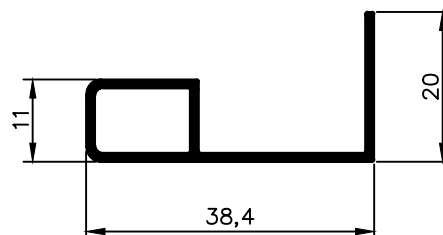
NX 6069 0,287 Kg/m
