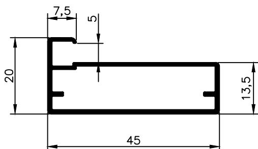
NX 5550 0,376 Kg/m
