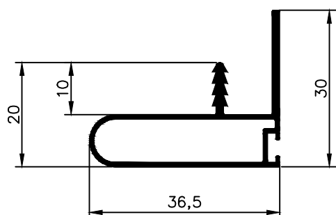
NX 2128 0,357 Kg/m
