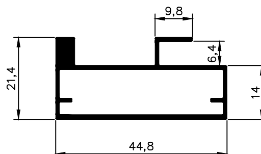
NX 3588 0,493 Kg/m
