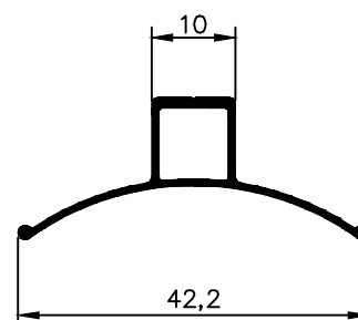
NX 4416 0,178 Kg/m
