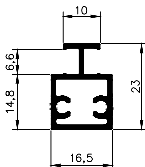
NX 2716 0,327 Kg/m
