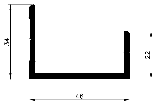
NX 4663 0,625 Kg/m
