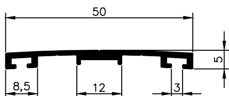
NX 2897 0,278 g/m
