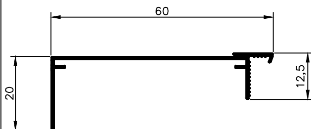
NX 4964 0,254 Kg/m
