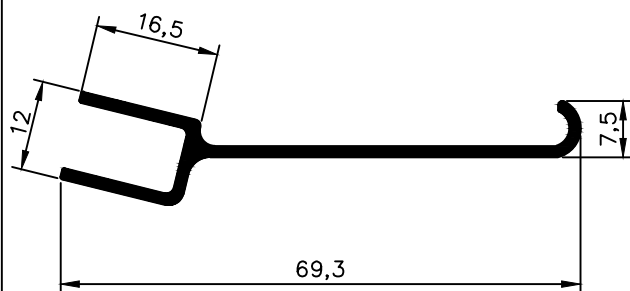
NX 2234 0,406 Kg/m
