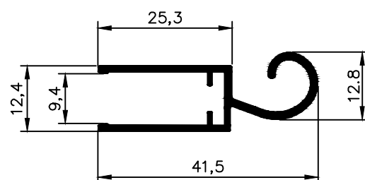
NX 2158 0,350 Kg/m
