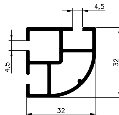
NX 0497 0,640 Kg/m
