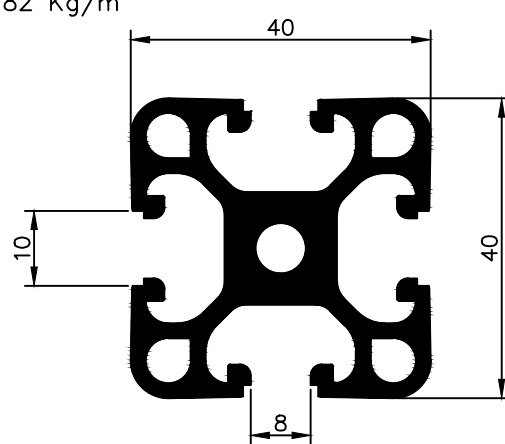
NX 0454 1,782 Kg/m
