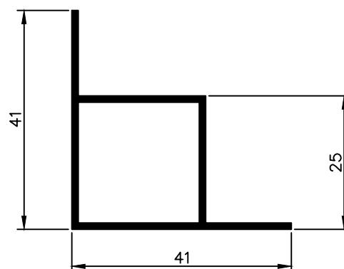
NX 1002 0,414 Kg/m
