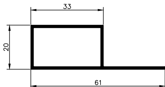
NX 4082 0,420 Kg/m
