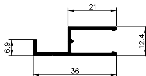
NX 2722 0,259 Kg/m
