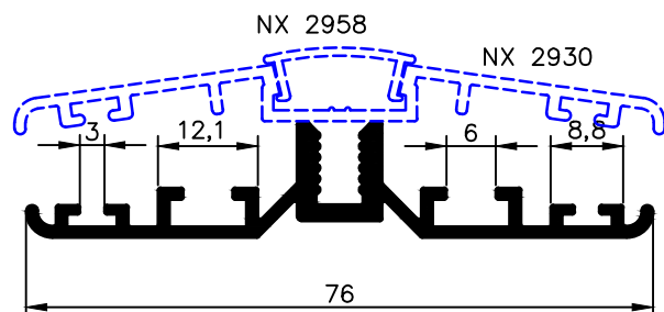
NX 3032 0,604 Kg/m
