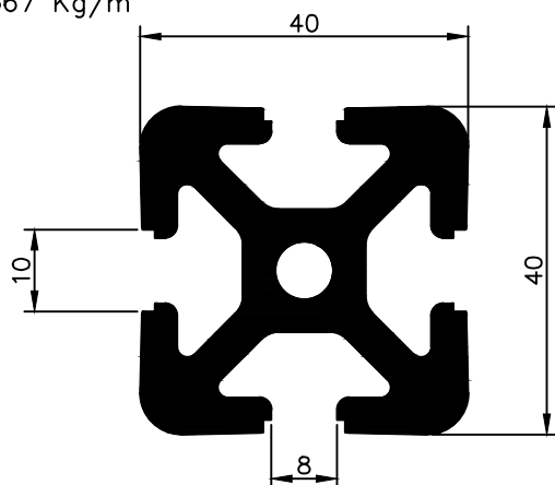
NX 0453 2,367 Kg/m
