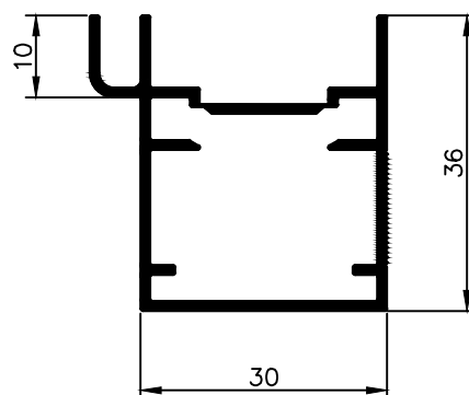
NX 3671 0,517 Kg/m
