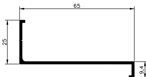
NX 6240 0,379 Kg/m
