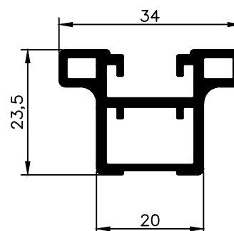
NX 4892 0,592 Kg/m
