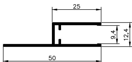
NX 2159 0,292 g/m
