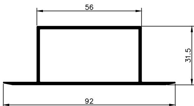
NX 3169 0,820 Kg/m
