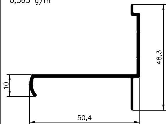
NX 2545 0,363 g/m
