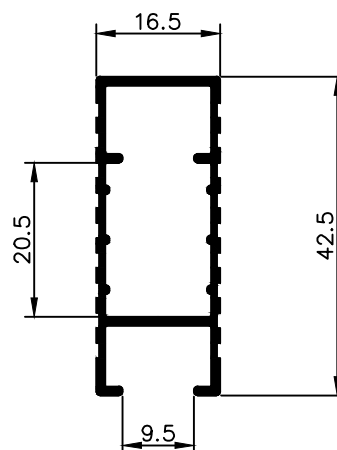
NX 1534 0,366 Kg/m
