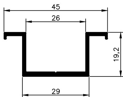
NX 6239 0,368 Kg/m
