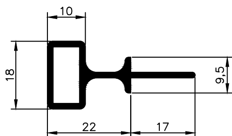
NX 0470 0,367 Kg/m
