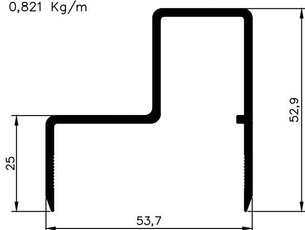
NX 5855 0,821 Kg/m
