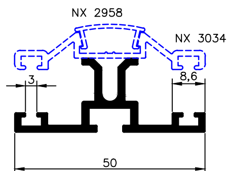
NX 3033 0,531 Kg/m
