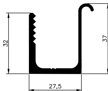
NX 0494 0,737 Kg/m
