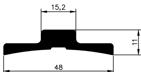
NX 5812 0,664 Kg/m
