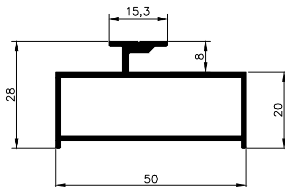
NX 0693 0,572 Kg/m
