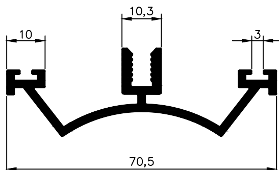
NX 3031 0,805 Kg/m
