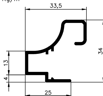
NX 0412 0,408 Kg/m
