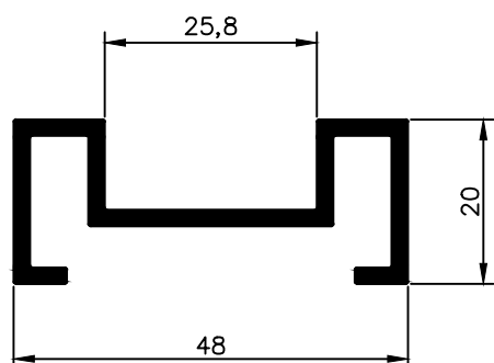
NX 5857 0,623 Kg/m
