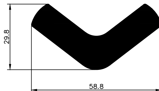
NX 0031 2,141 Kg/m
