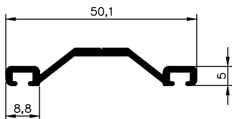
NX 2931 0,311 Kg/m
