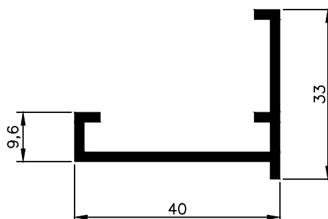
NX 0399 0,454 Kg/m
