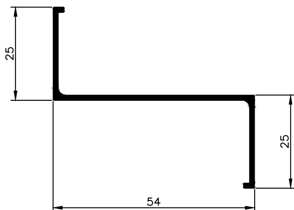
NX 2132 0,400 Kg/m
