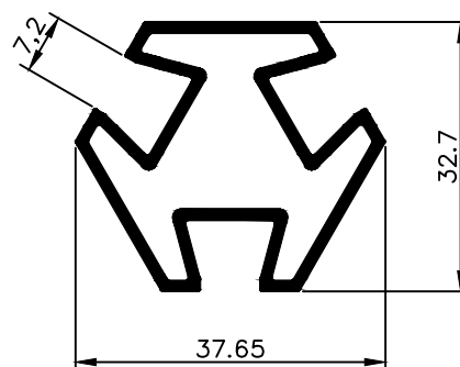
NX 0452 0,653 Kg/m
