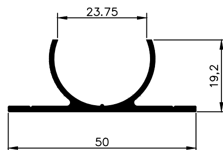
NX 3397 0,358 Kg/m
