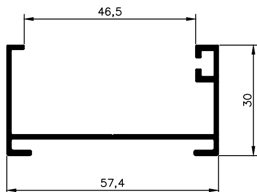
NX 4887 0,486 Kg/m
