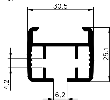
NX 5583 0,500 Kg/m
