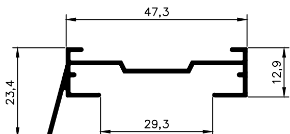
NX 3658 0,319 Kg/m
