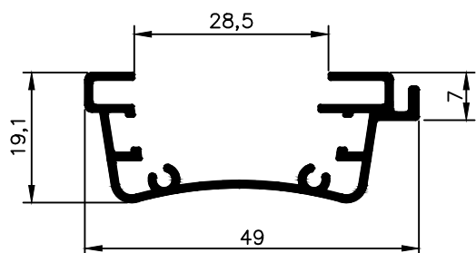
NX 1957 0,411 Kg/m
