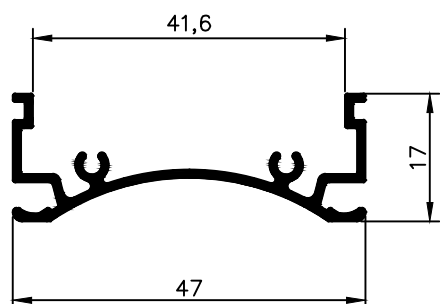
NX 4051 0,349 Kg/m
