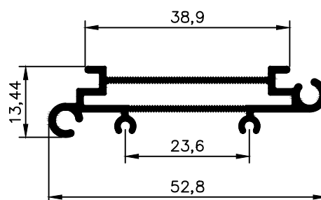
NX 5372 0,418 Kg/m
