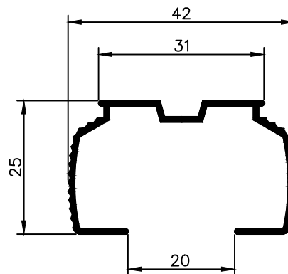
NX 0642 0,291 Kg/m
