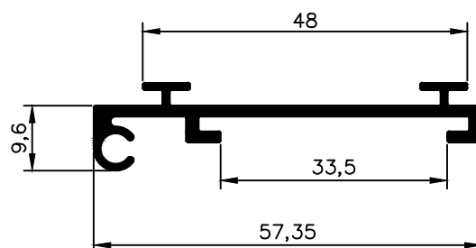
NX 4587 0,344 Kg/m
