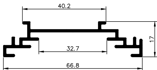
NX 1722 0,488 Kg/m
