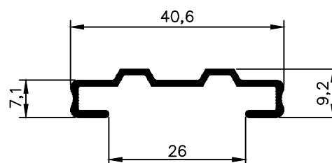
NX 3458 0,222 Kg/m
