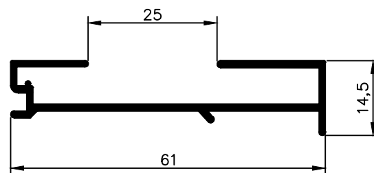
NX 1368 0,436 Kg/m
