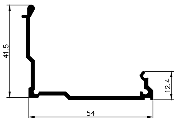
NX 1117 0,461 Kg/m
