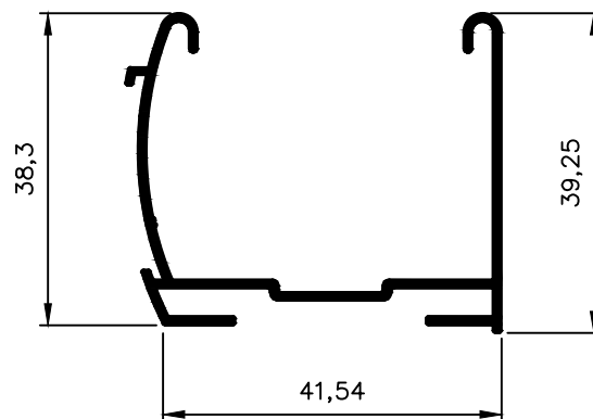
NX 6242 0,462 Kg/m
