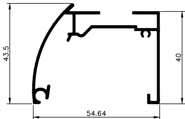
NX 3450 0,612 Kg/m
