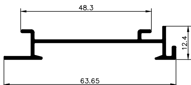
NX 1605 0,338 Kg/m
