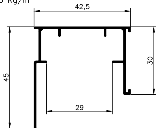
NX 5995 0,335 Kg/m
