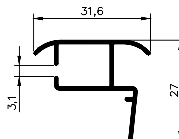
NX 4593 0,243 Kg/m
