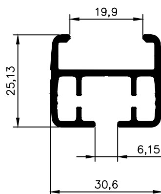
NX 6198 0,512 Kg/m
