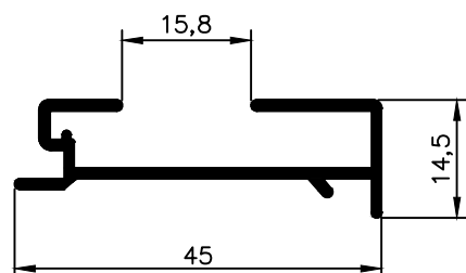
NX 1343 0,344 Kg/m
