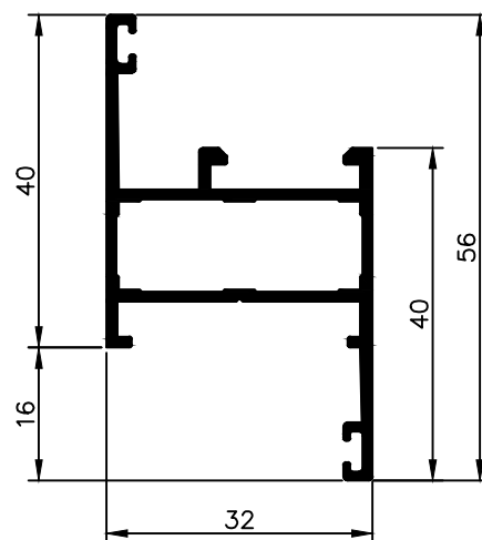
SC-6155 0,589 kg/m
