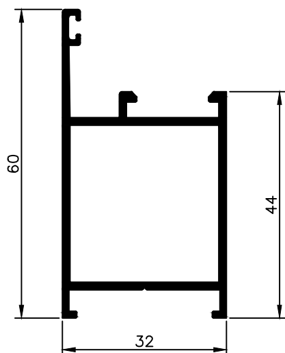
SC-6156 0,715 kg/m
