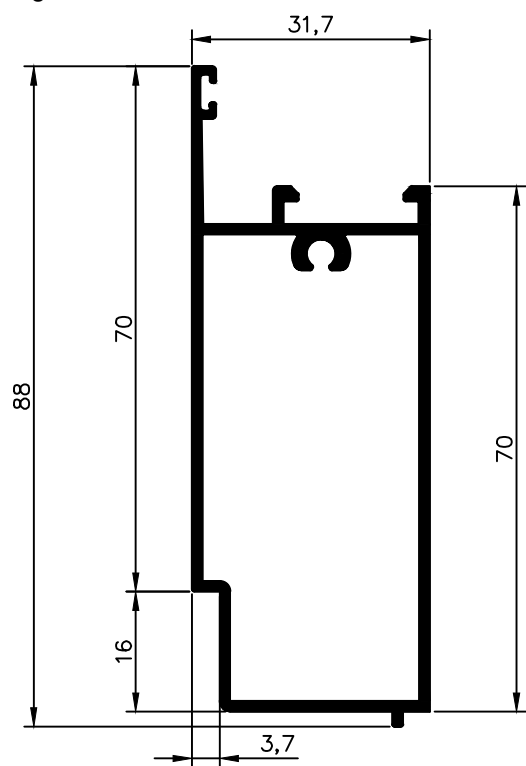
SC-6166 0,934 kg/m
