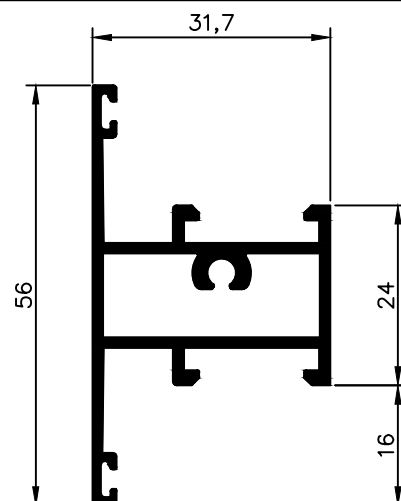
SC-6161 0,695 kg/m
