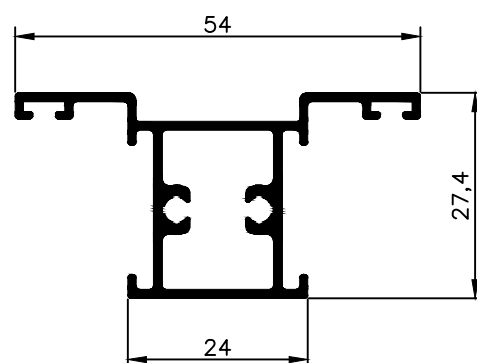
NX 2633 0,552 kg/m
