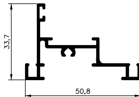
NX 3367 0,459 kg/m
