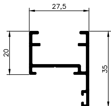
NX 5511 0,366 kg/m
