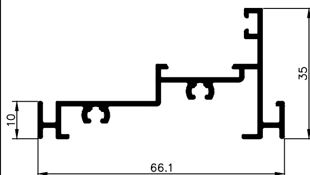
NX 0608 0,605 kg/m
