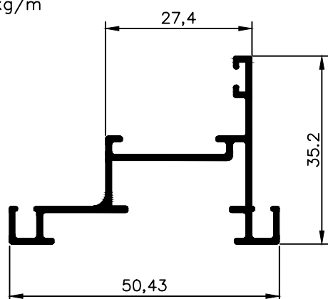
NX 2666 0,452 kg/m
