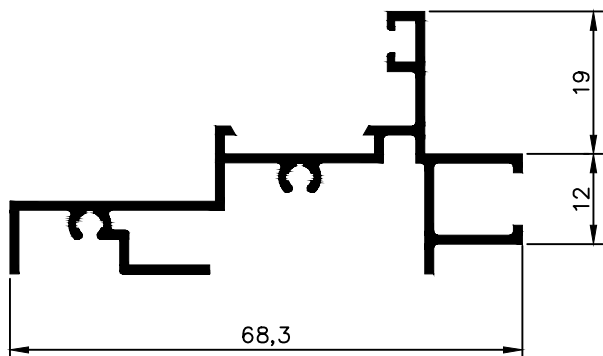
NX 1207 0,645 kg/m
