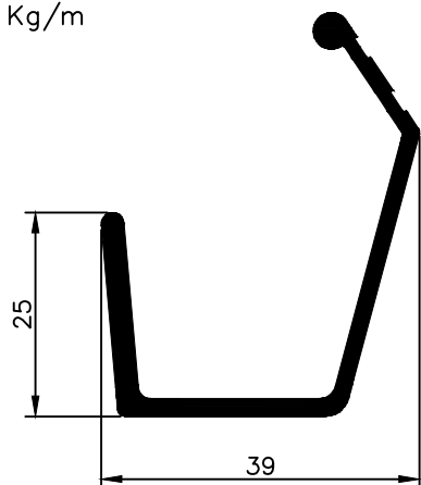
NX 3785 0,634 Kg/m
