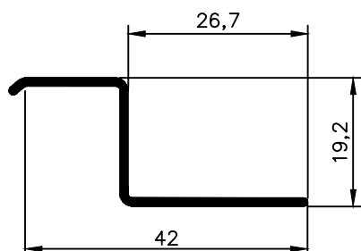
NX 1908 0,217 Kg/m
