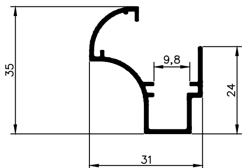
NX 2063 0,322 Kg/m
