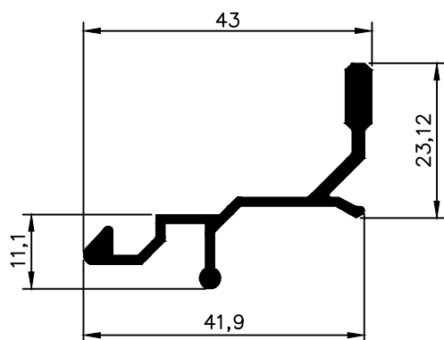
NX 1179 0,431 Kg/m
