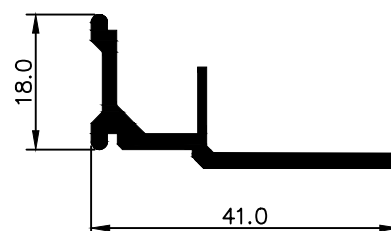
NX 0225 0,372 Kg/m
