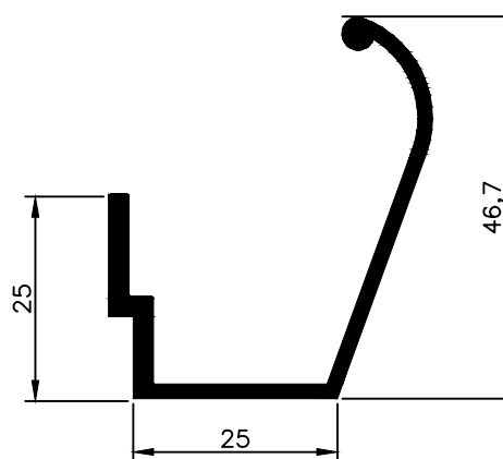
NX 1992 0,566Kg/m
