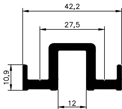
NX 0996 0,861 Kg/m
