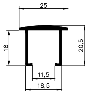
NX 2965 0,271 Kg/m
