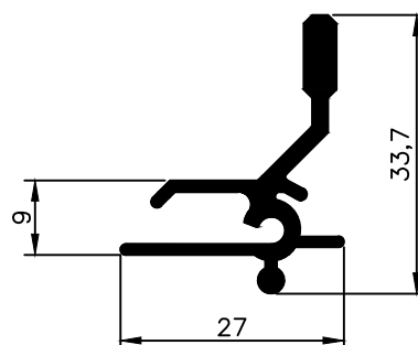
NX 1181 0,426 Kg/m
