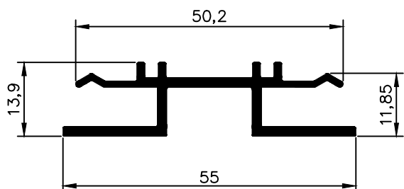
NX 2660 0,521 Kg/m
