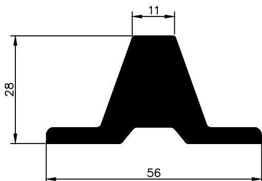
NX 3612 1,737 Kg/m
