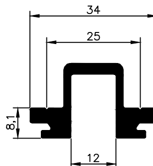
NX 0997 0,609 Kg/m
