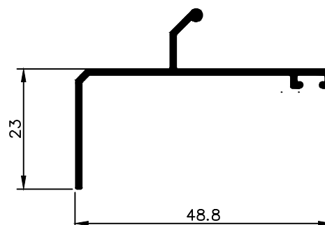
NX 0109 0,294 Kg/m
