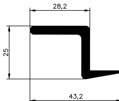
NX 2964 0,621 Kg/m
