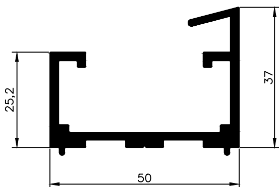
NX 5073 0,973 Kg/m
