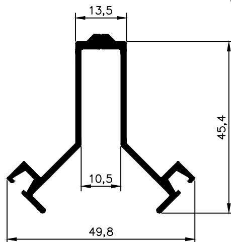
NX 2331 0,627 Kg/m
