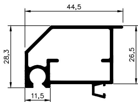
NX 2196 0,648 Kg/m
