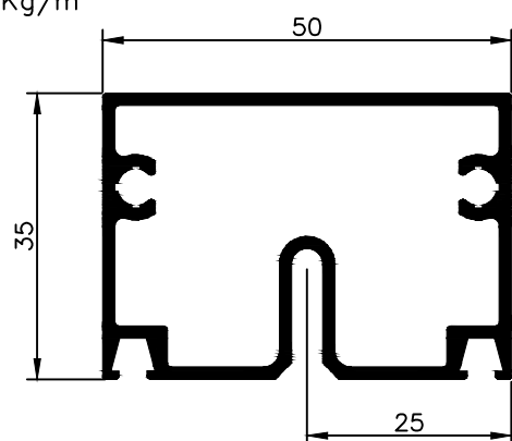
NX 2199 0,951 Kg/m
