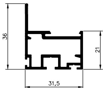
NX 5434 (Desenvolvido pela FISE) 0,554 Kg/m
