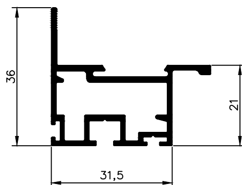
NX 5564 (Desenvolvido pela FISE) 0,599 Kg/m
