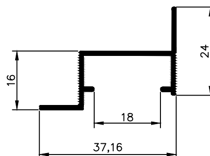
NX 2456 0,256 Kg/m
