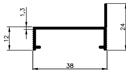
NX 0887 0,276 Kg/m
