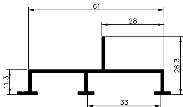
NX 0588 0,473 Kg/m
