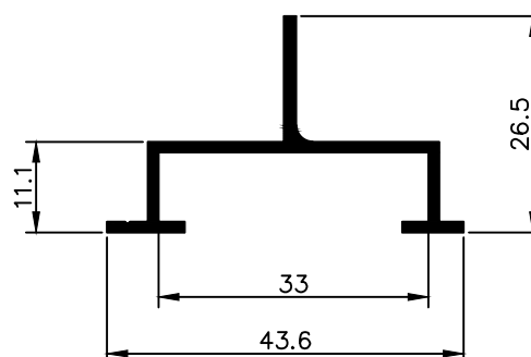
NX 0206 0,306 Kg/m
